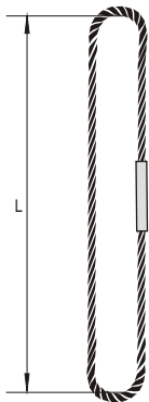
Cablu de legatura inelar cu manson presat, mat sau zinacat
